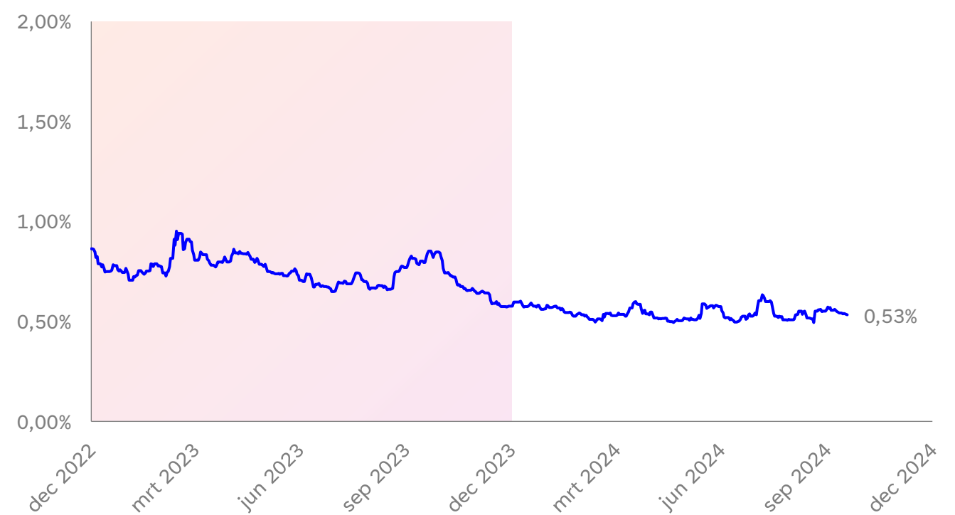
Figuur 2: Kredietrisico
