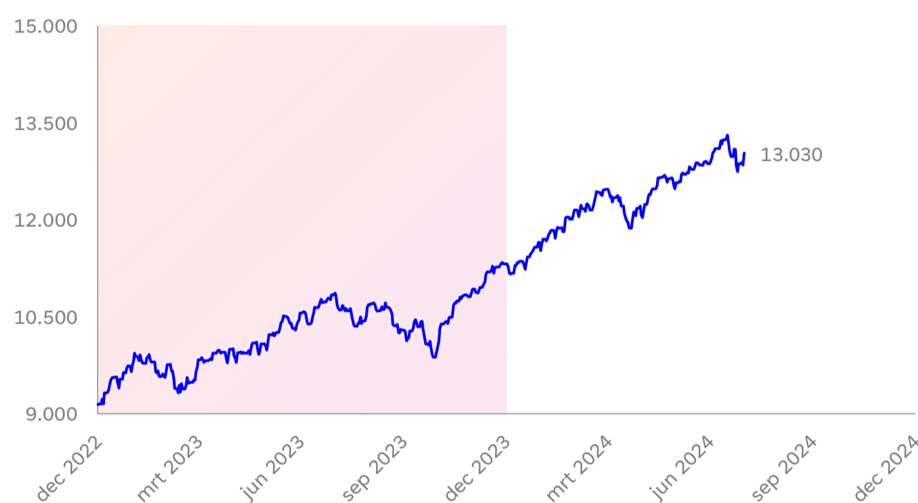
Figuur 4: Aandelenrisico
